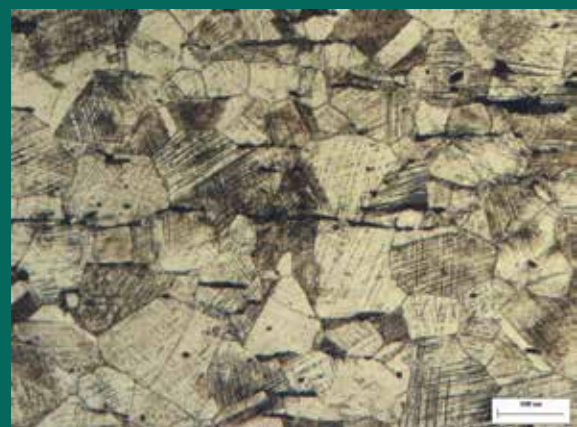
▲ โครงสร้างจุลภาคแสดงให้เห็นแถบการเลื่อน (slip bands) ปริมาณมากบริเวณใกล้ผิวด้านนอกของท่อ
