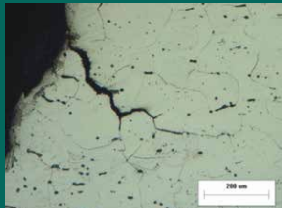
▲ โครงสร้างมหภาคแสดงให้เห็นรอยแตกขยาดตามขอบเกรน
